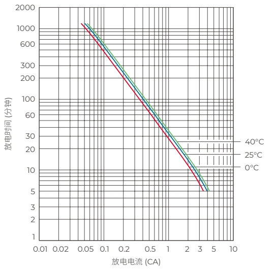
放电电流与放电时间关系曲线
