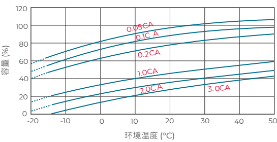
环境温度与放电容量的关系
