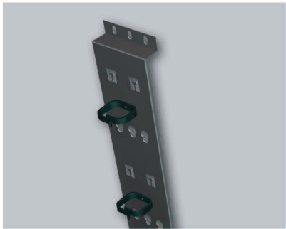
垂直理线通道 (标配) +理线圈 (选配)
